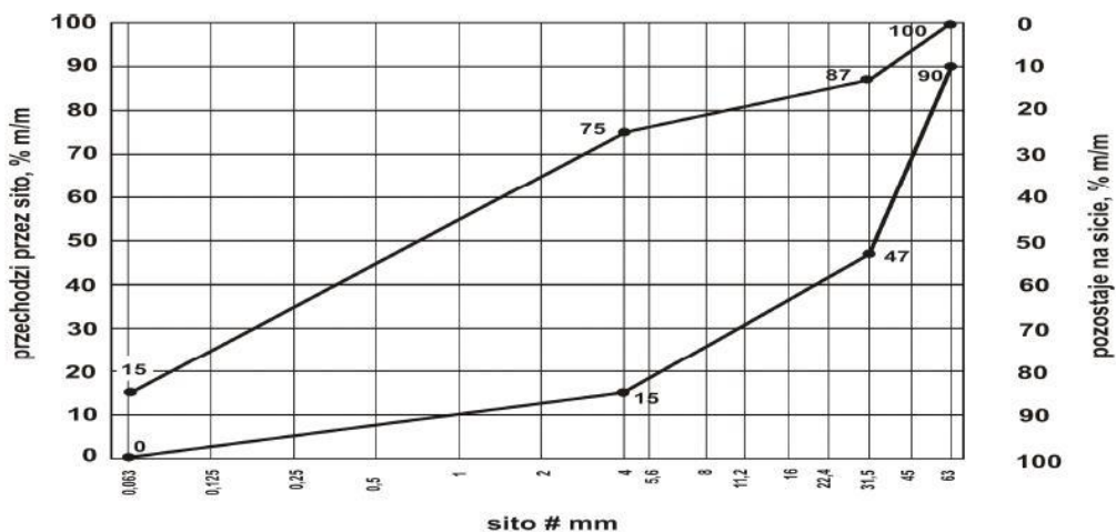
Rys.2. Mieszanka niezwiązana 0/63 mm do warstwy ulepszonego podłoża
