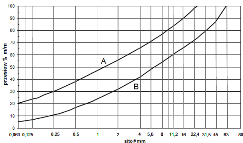
Rys. 5.1. Krzywe graniczne uziarnienia mieszanki mineralno-cementowej do warstwy podbudowy z mieszanki MCE
